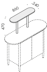
Shelf with with rovere massello wood veneer supports / Étagère avec supports en bois massif rovere massello / Regal mit Rovere Massello Holzfurnier Unterstützt
