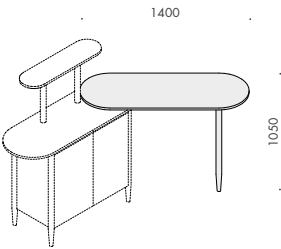
Side top with rovere massello wood veneer leg / Plateau lateral avec pied en bois massif rovere massello Seitenetische mit Rovere Massello Holzfurnier Beine
